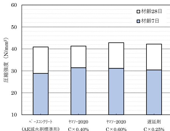
圧縮強度
