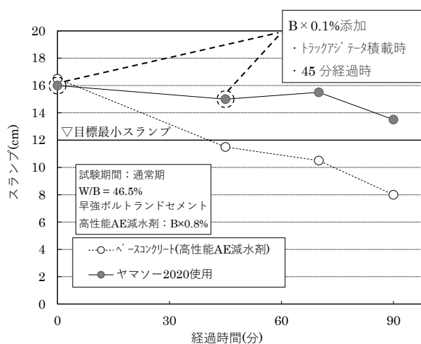
分割添加におけるスランプの経時変化【実機】
