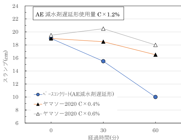
環境温度 38°Cにおけるスランプの経時変化【室内】
