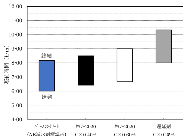
凝結時間
