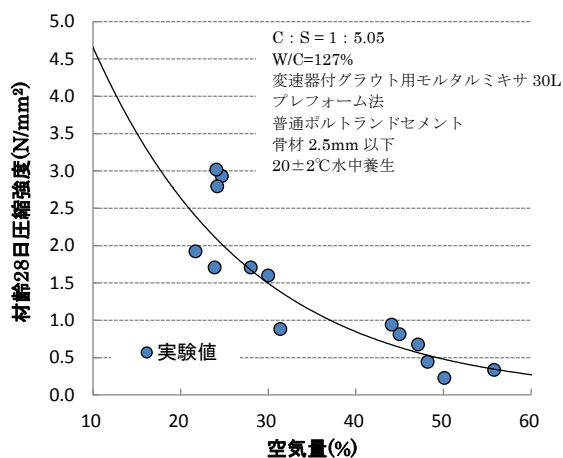
図-4 空気量と材齢 28 日圧縮強度の関係
