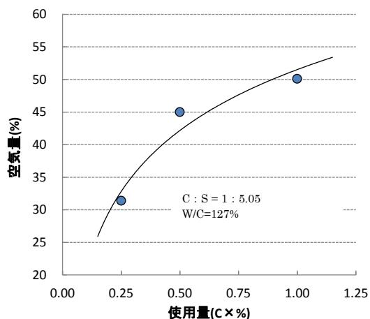
図-1 使用量と空気量の関係
