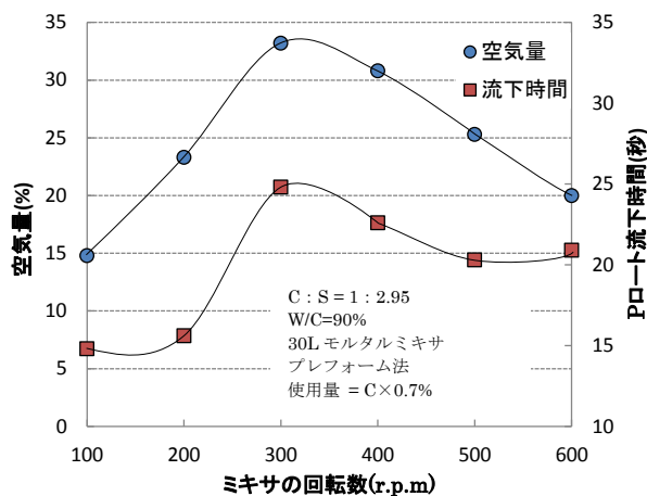
図-2 ミキサの回転数と空気量及びPポート流下時間の関係
