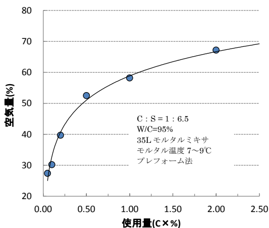
図-3 防水押えモルタル用試験による使用量と空気量の関係
