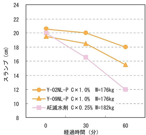
経過時間とスランプの関係(W/C=57.5%)
