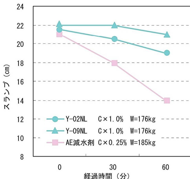
経過時間とスランプの関係(W/C=47.5%)
