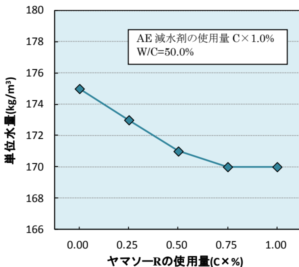
図1 使用量と単位水量の関係
