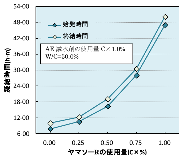
図2 使用量と凝結時間の関係
