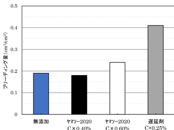
ブリーディング量
