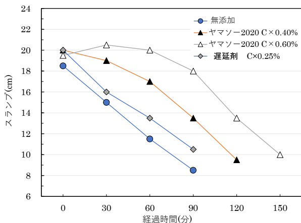
スランプの経時変化
